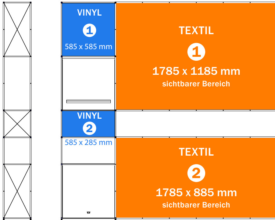
FRONT ANSICHT
